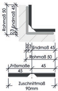
Innenecke
