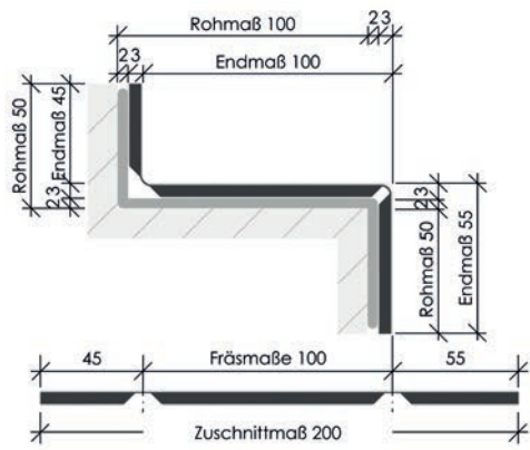
Brüstung
