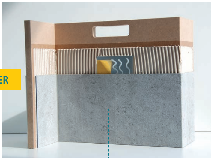
Fugenloser Plattenstoß
