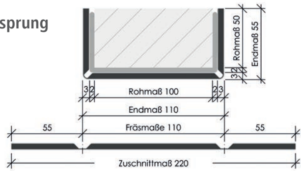
Außenecke
