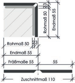
Außenecke
